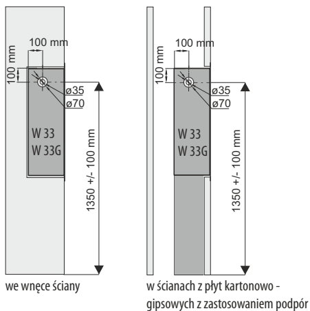
Rys. 2 Hydrant wnętkowy
