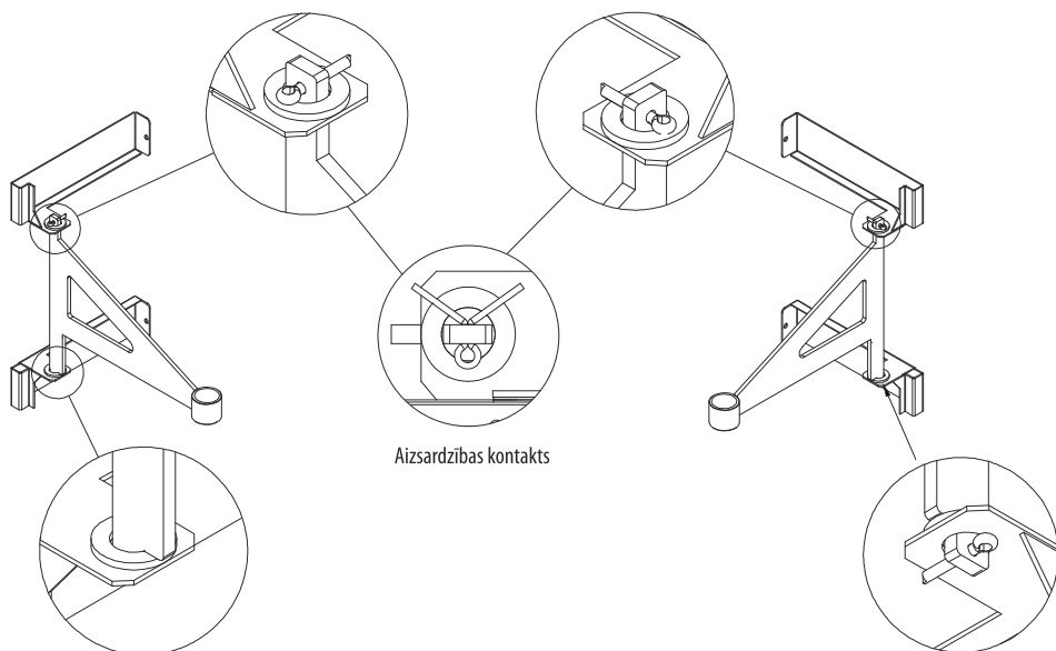
1. attēls. Savienotāja atrašanās vieta kreisajā pusē
