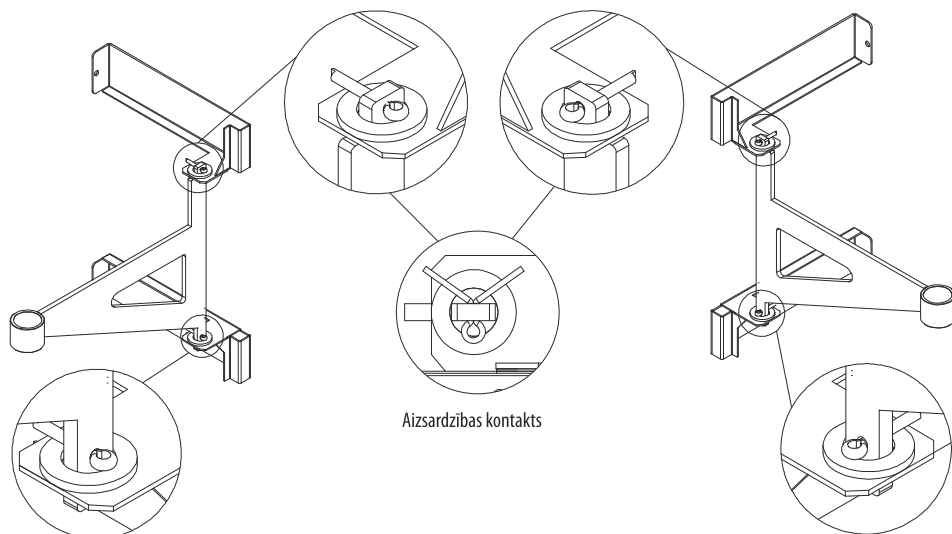
3 att. Savienojuma vieta kreisajā pusē
