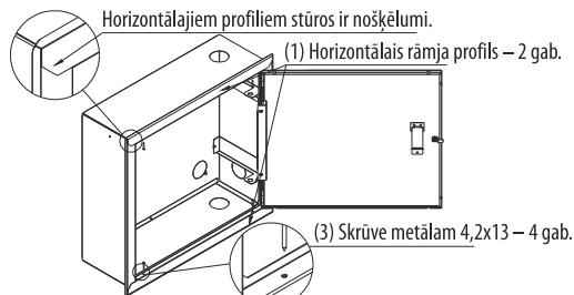
2. att. Horizontālo rāmja profilu uzstādīšana
