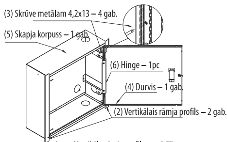
1. att. Vertikālo rāmja profilu uzstādīšana
