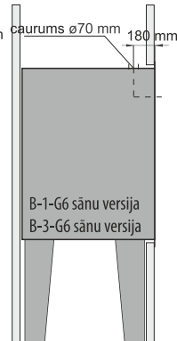
2. attēls. Iebūvētie (nišas) hidranti
