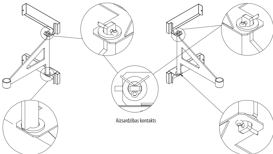
3. attēls. Savienotāja atrašanās vieta kreisajā
