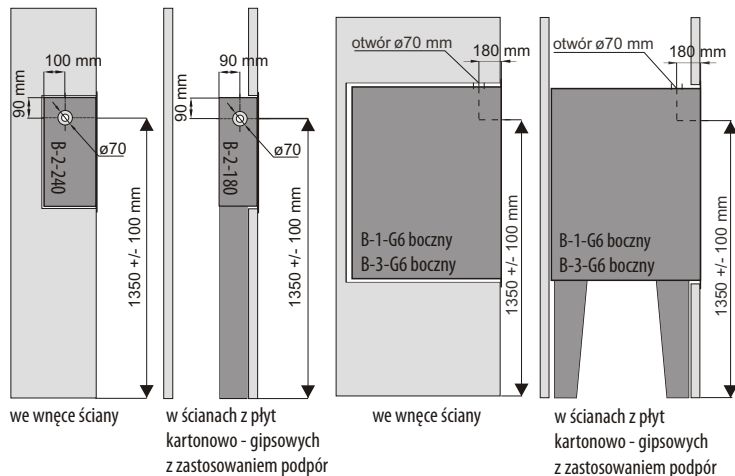
Rys. 2 Hydrant wężkowy
