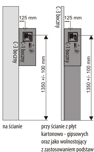
Rys. 1 Hydrant zawieszany
