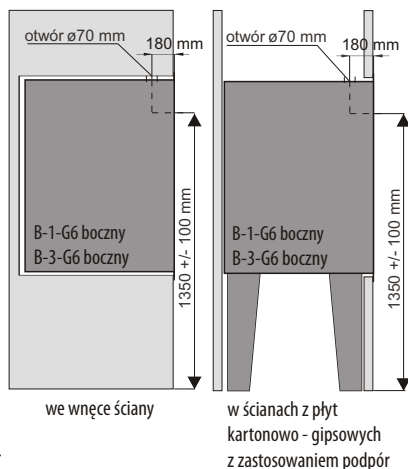
Rys. 2 Hydrant wężkowy
