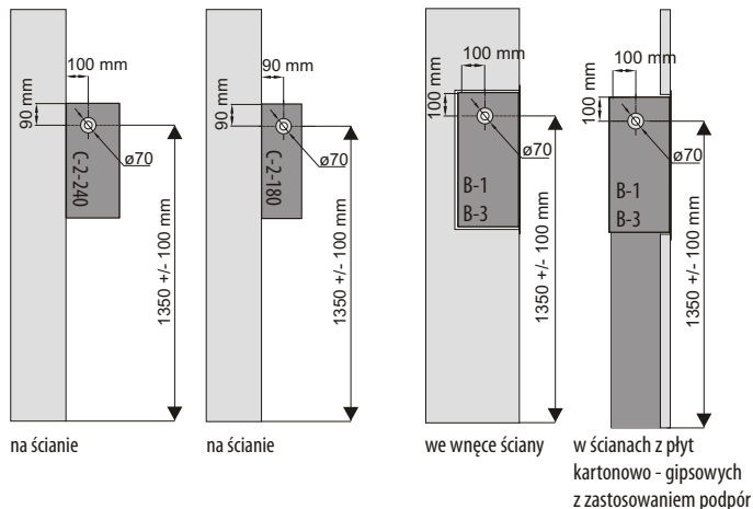
Rys. 2 Hydrant wężkowy
